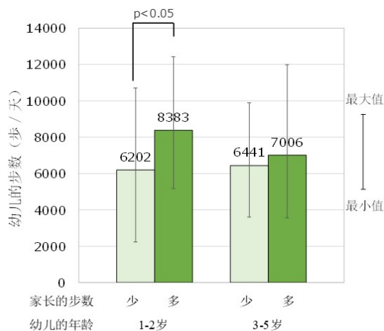
图4 家长与幼儿的步数
