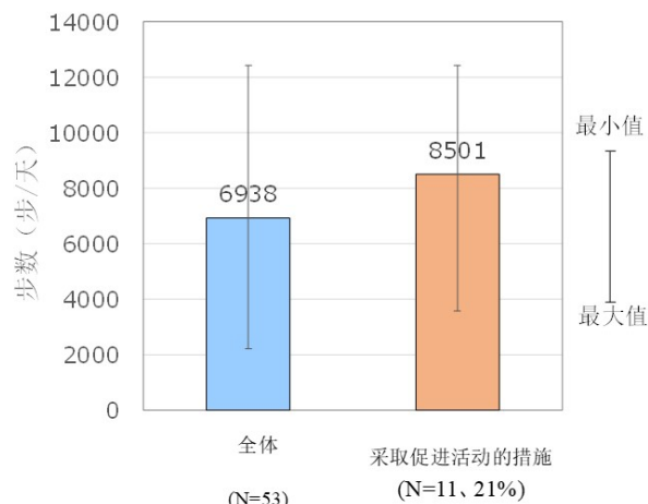
图3 没有外出但采取促进活动的措施时幼儿的步数
