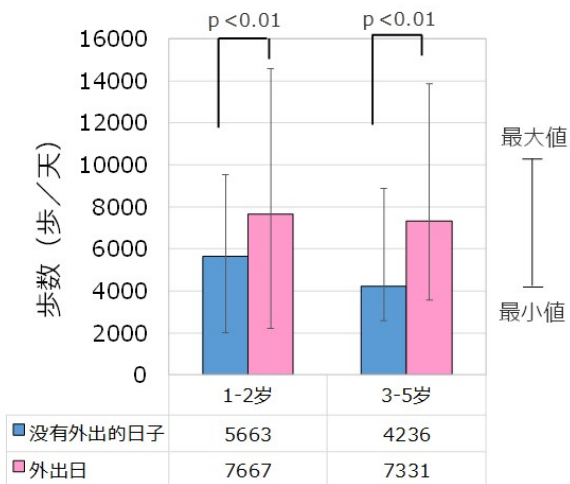
图2 外出与否和幼儿步数
