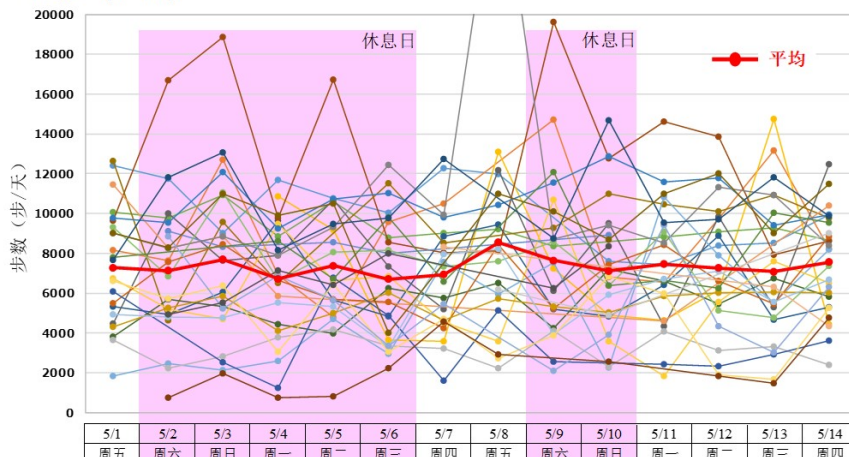
图1 调查期间幼儿的每日步数
